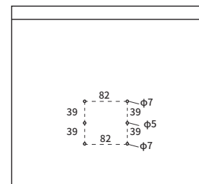
【本体背面 取付穴間隔】
