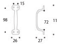
G620767 ※ ハンドル CN スクエア AN 1,250円 (税込1,375円) サイズ/約w112 × d27 × h26mm 素材/真鍮古色仕上げ ※ビス付
