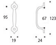
G620765 ※ ハンドル CN オーバル AN 1,200円 (税込1,320円) サイズ/約w123 × d24 × h19mm 素材/真鍮古色仕上げ ※ビス付
