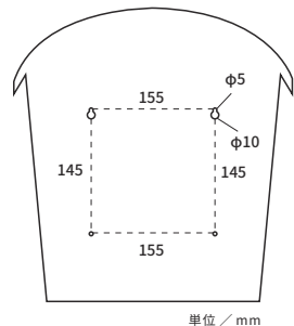
【本体背面 取付穴間隔】
