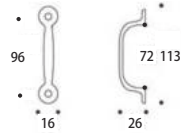
G620766 ※ ハンドル CN ラウンド AN 1,200円 (税込1,320円) サイズ/約w113 × d26 × h16mm 素材/真鍮古色仕上げ ※ビス付
